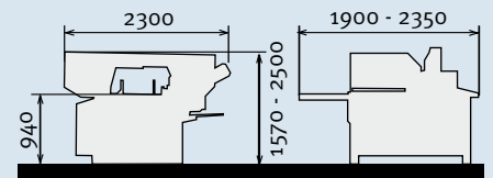
Abmessung BMBS 350 x 400 CNC-DG-F
