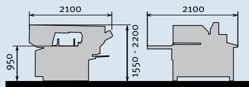
Abmessung BMBS 290 x 290 CNC-F
